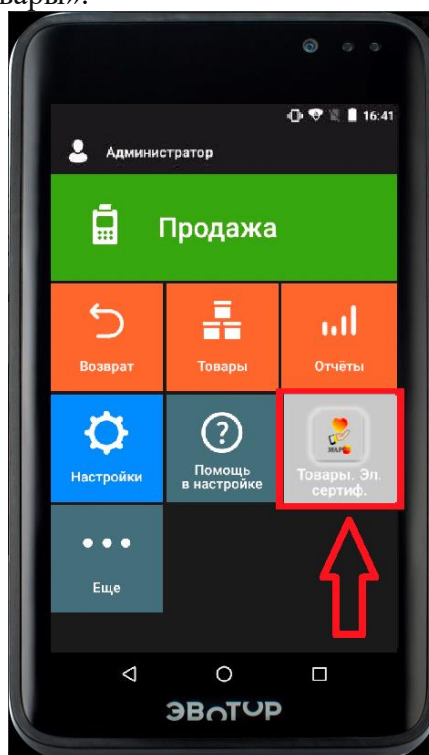
Рисунок 1– Главное окно
