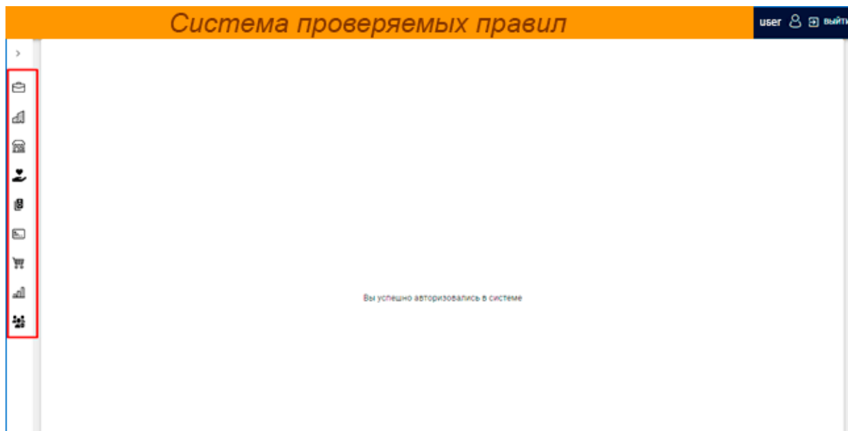
Рисунок 1. Главное окно
